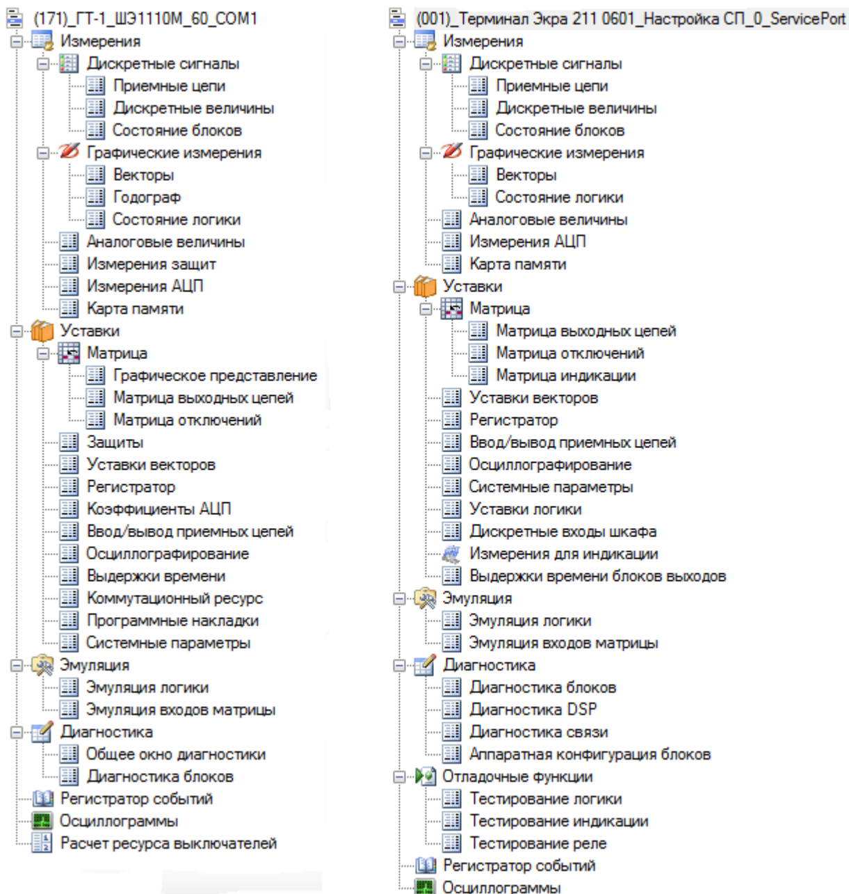
Рисунок 2.11 - Меню терминала (слева – 100-й серии, справа – 200-й серии)
