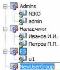
Рисунок 4.7 - Добавление группы
